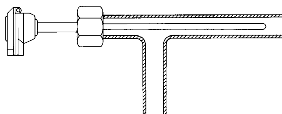
配管パイプ取付
