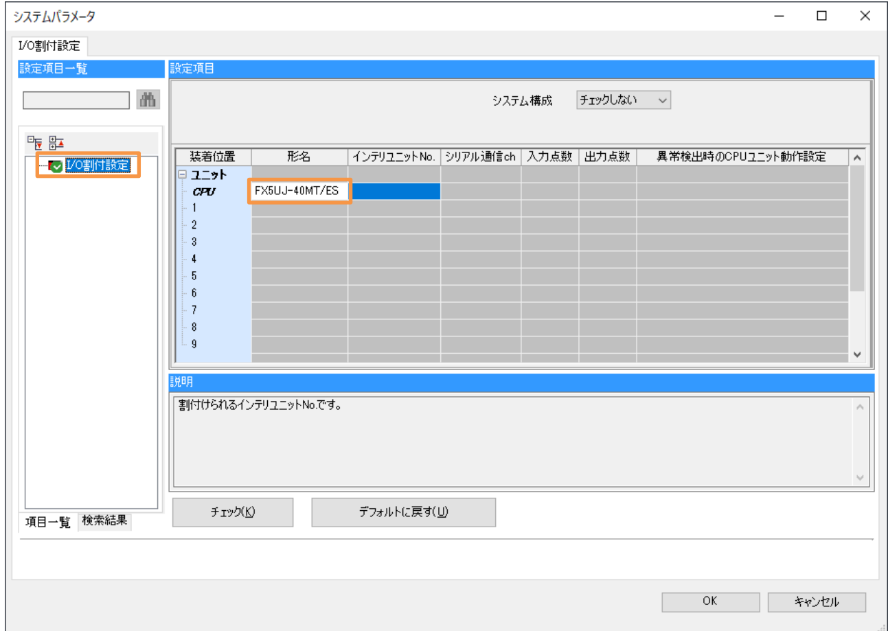
図 7-2I/O 割付設定
