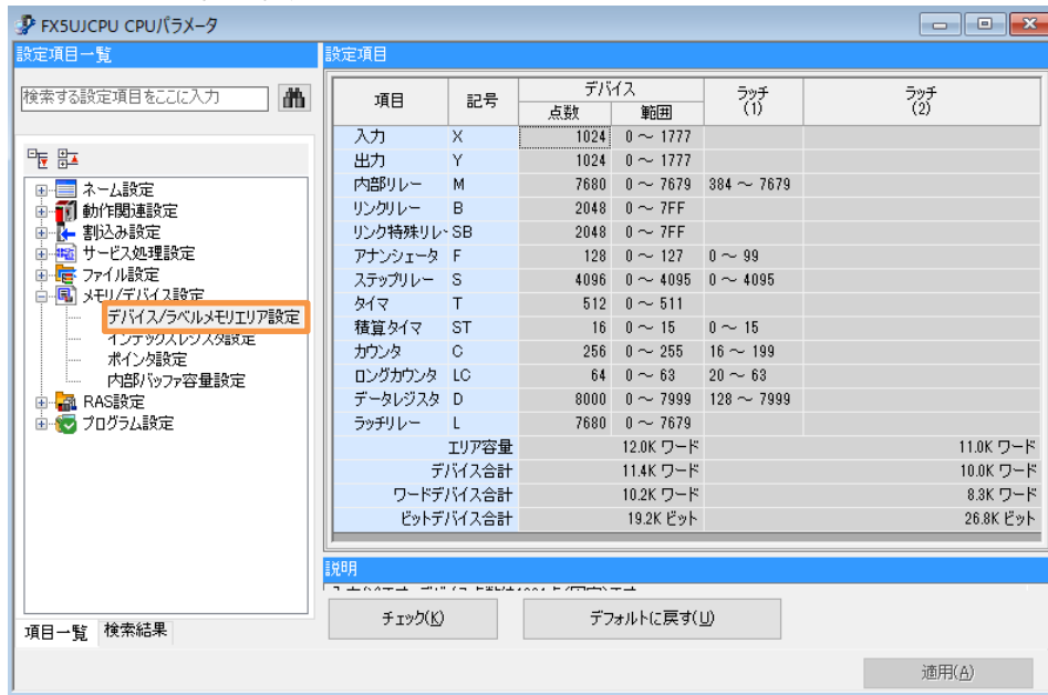
図 7-3 デバイス(高速)設定図
