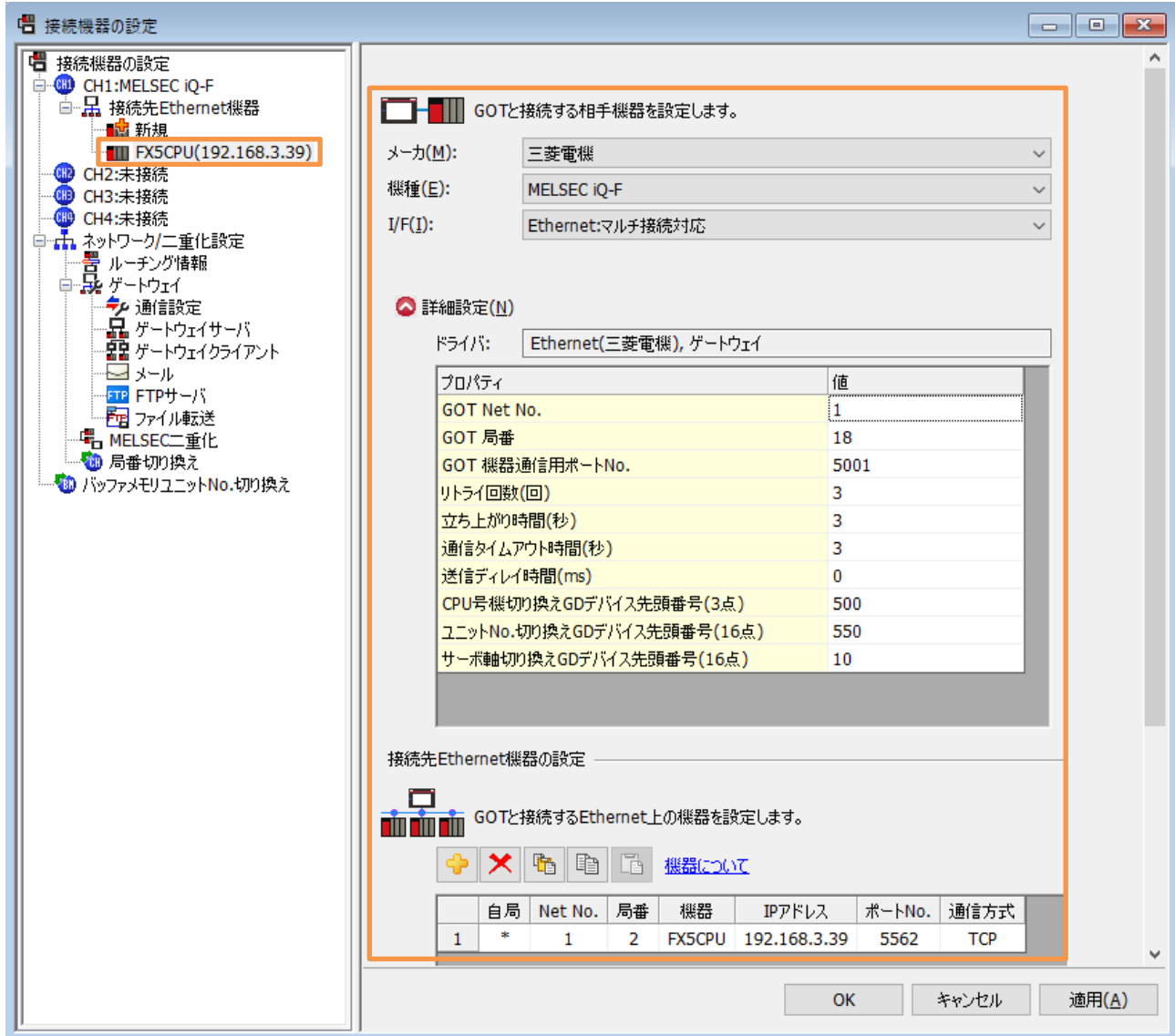
図 10-5 接続機器の設定
