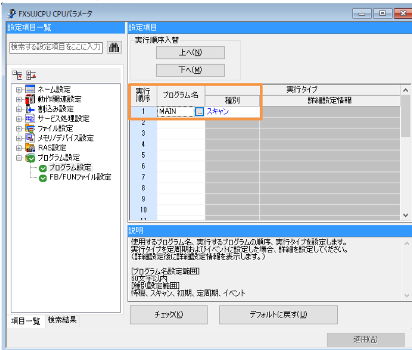
図 7-5 プログラム設定詳細
